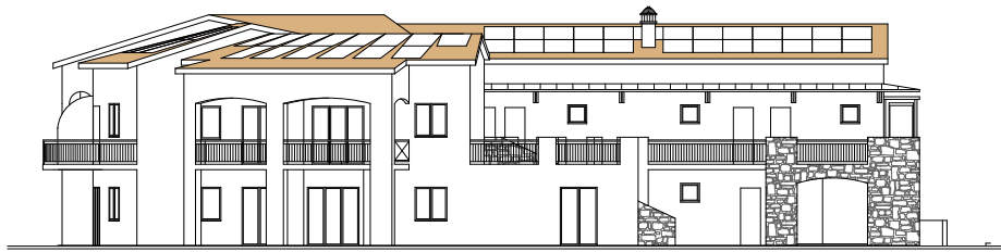
Prospetto Est di progetto
